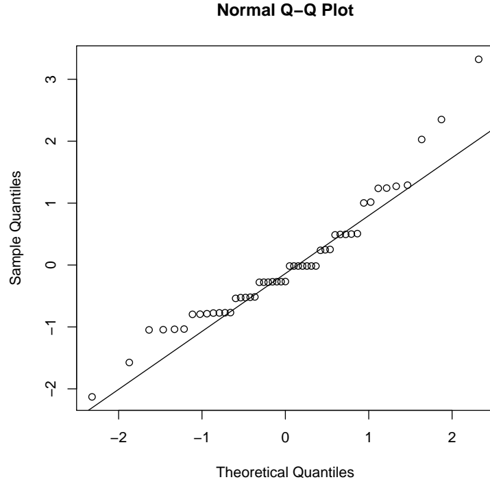
FIGURE 9.3: Graphique Quantile-Quantile
